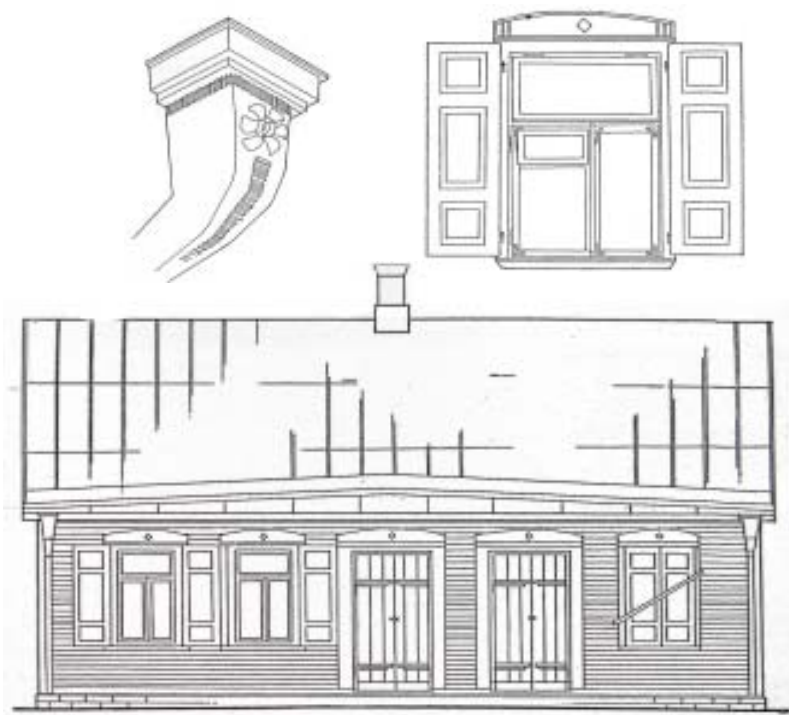
Vytauto g. 7 namo fasado, lietvamzdžio detalės ir lango brėžiniai.
