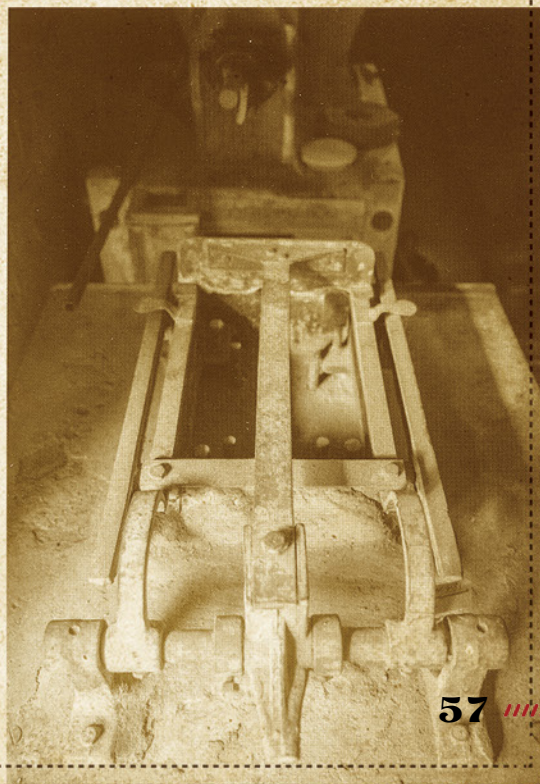
Margelių čerpių gamybos mašina. Naudota 1938 m.
